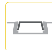
K23 P20 max. 11mm
