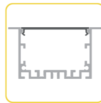
KN30 P36 max. 39mm
