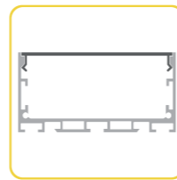
KN28 P36 max. 64mm
