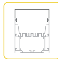
KN43 P38 max. 54mm
