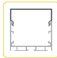
KN25 P35 max. 39mm
