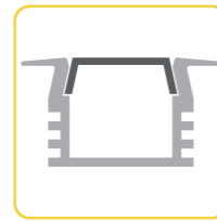
K25 P20 max. 11mm
