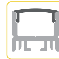
K53 P22 max. 13mm
